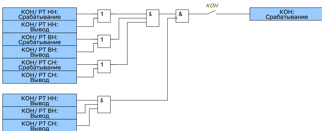
Рисунок 2.17 – Функциональная схема логики КОН
